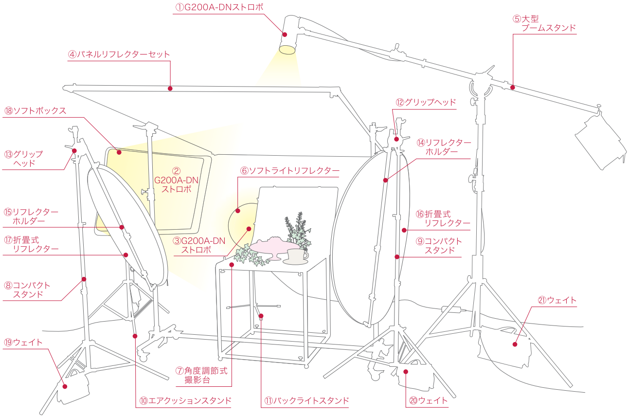
撮影機材セットアップ構成例
