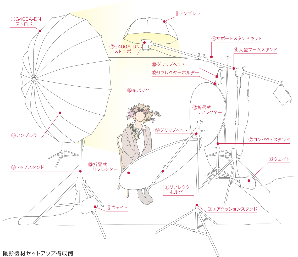
撮影機材セットアップ構成例
